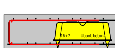
Dettaglio 8 - Armatura di bordo: forchetta
