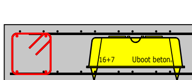
Dettaglio 7 - Armatura di bordo: cordolo
